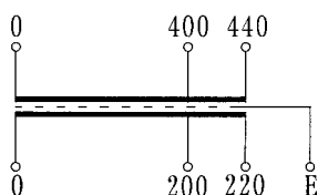
結線図
