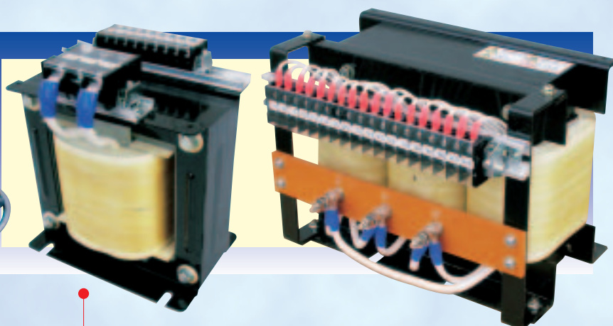
充電器用トランス
