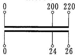
結線図
