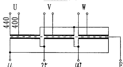
結線図
