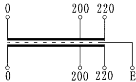
結線図
